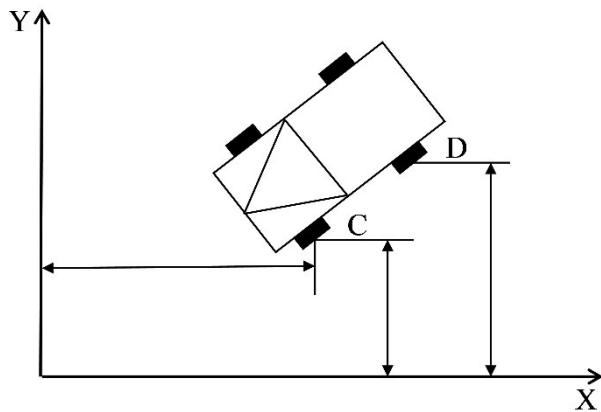
Рис. 10. Принципи графічної фіксації транспортних засобів та інших слідів ДТП у прямокутній системі координат
